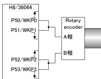
図. 6.8: ロータリエンコーダ1つを4通倍カウントする場合の接続例
