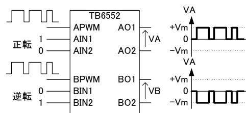
図. 5.6: PWM 信号と出力電圧の関係
