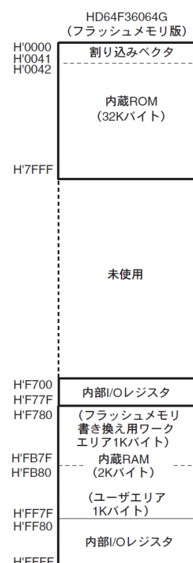
図 2.3: メモリマップ (Renesas H8/36064 ハードウェアマニュアルより)
