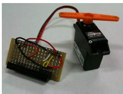
図. 5.7: RC サーボと接続用回路
