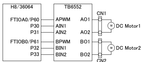
図. 5.5: マイコンとドライバ, モータの接続関係
