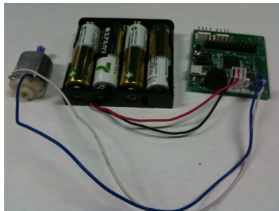
図. 5.1: DCモータと電池ボックスの接続
