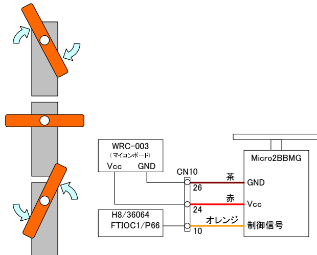
図. 5.10: マイコンボードと RC サーボの接続
