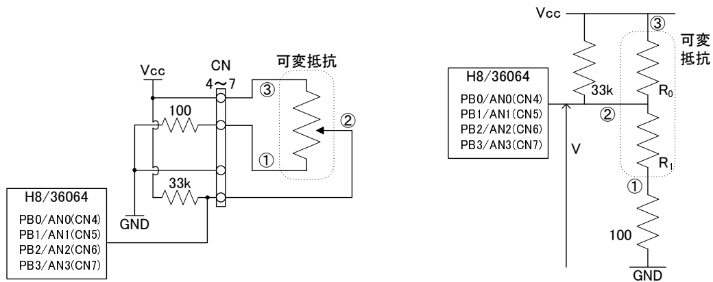
図. 6.1: 可変抵抗とその接続
