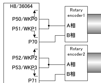
図. 6.9: ロータリエンコーダ2つを2通倍カウントする場合の接続例
