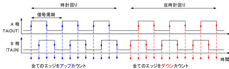
図. 6.7: ロータリエンコードの A 相/B 相出力と回転方向識別
