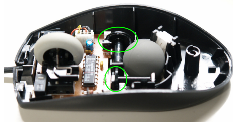
図. 6.5: ボール式マウスの中のロータリエンコード
