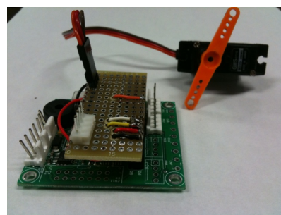
図. 5.8: RC サーボの接続
