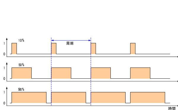
図. 5.2: PWMの例
